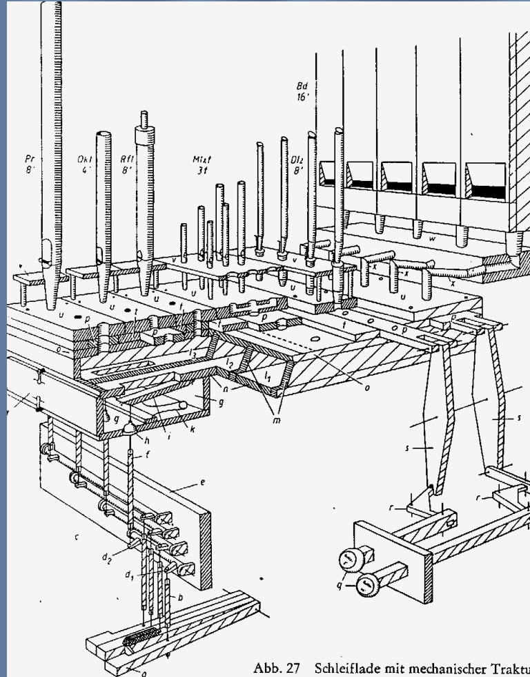
Abb. 27 Schleiflade mit mechanischer Traktur
